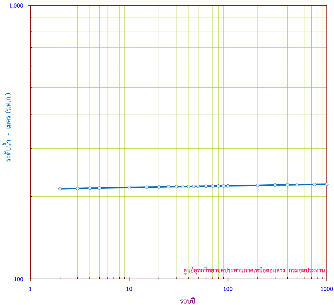
กราฟแสดง ระดับน้ำสูงสุดรายปี ขนาดรอบปีต่างๆ สถานี N.58 บ.กกม่วง อ.นครไทย จ.พิษณุโลก
